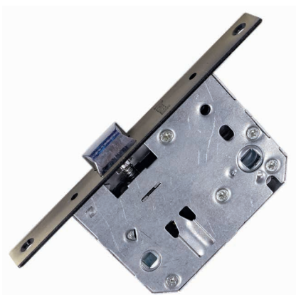
Защелка сантехническая A=70мм
